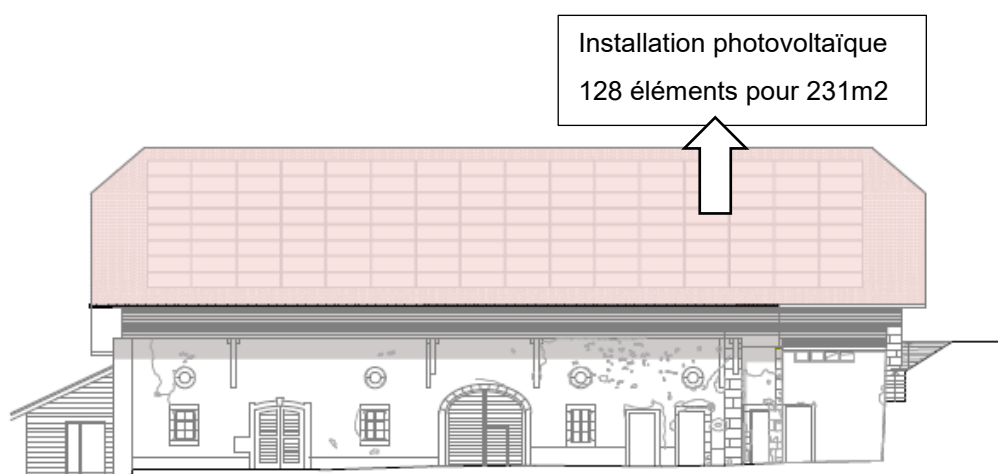
Façade Nord
