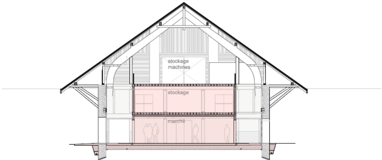
Coupe cc
