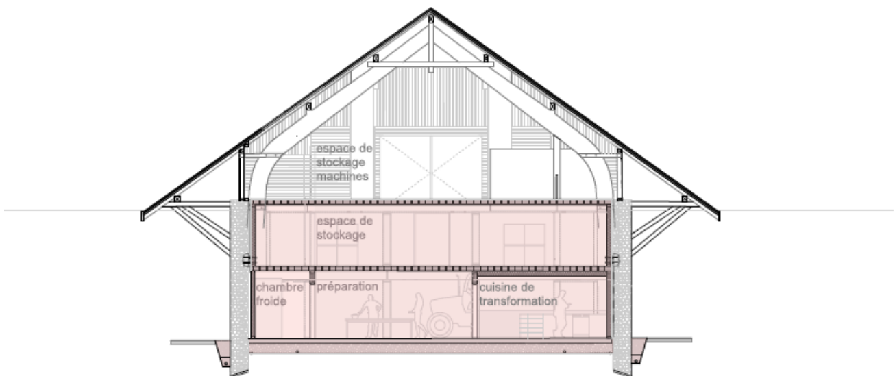
Coupe dd
