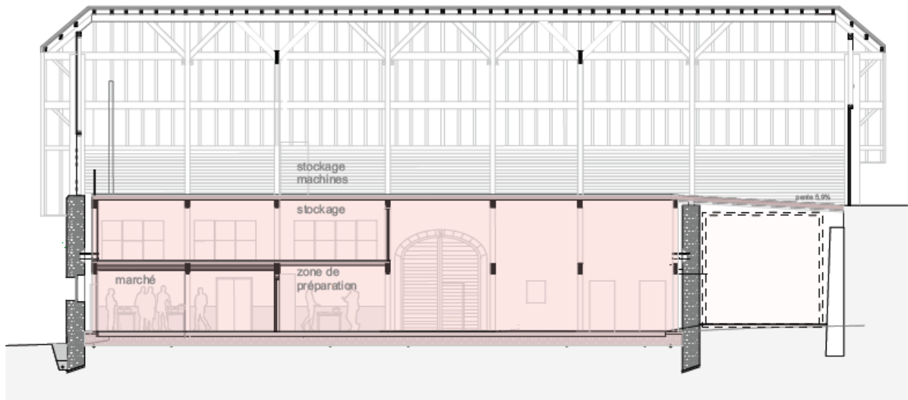
Coupe aa
